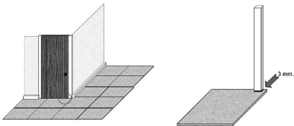
Encuentros con sectores singulares sin guardapolvos ni junquillos
