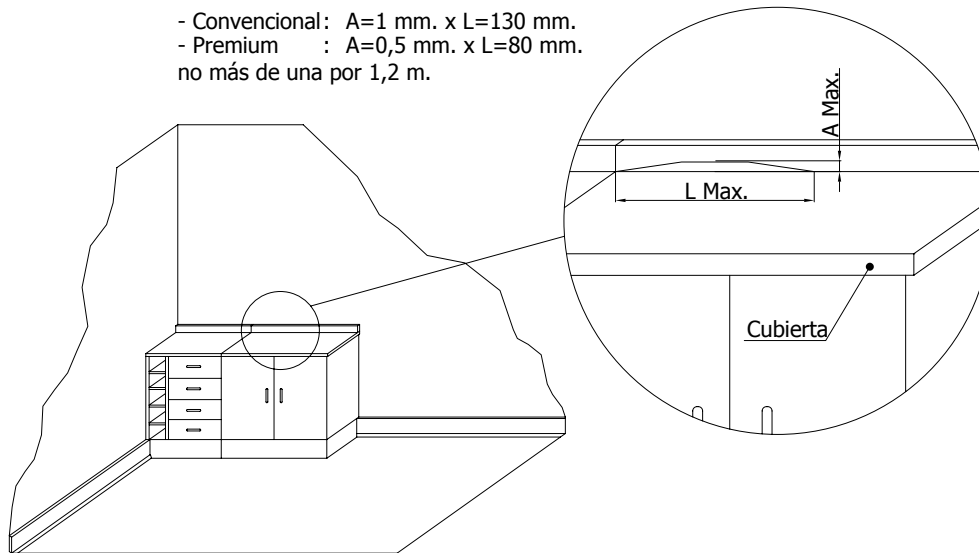
Espacio a la vista en mueble sin continuidad funcional.
